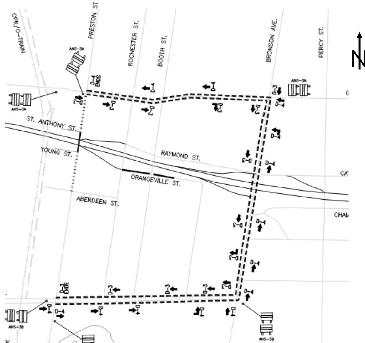
Figure 2 Fermeture itinéraire de déviation des véhicules de la rue Preston
