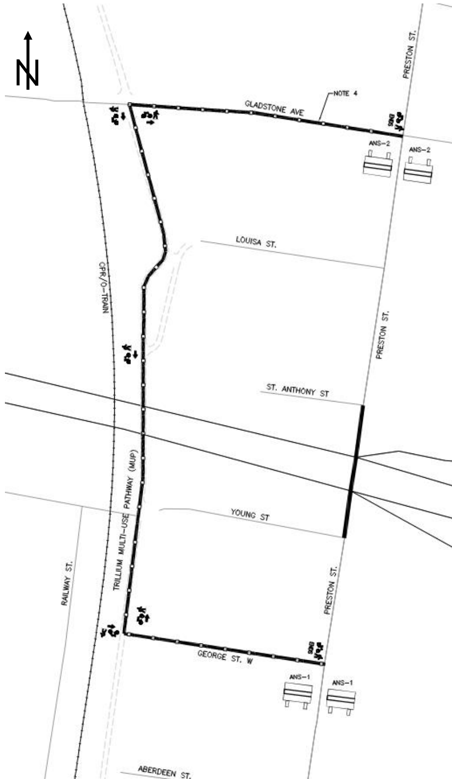
Figure 3 Fermeture itinéraire de déviation des piétons et cyclistes de la rue Preston
